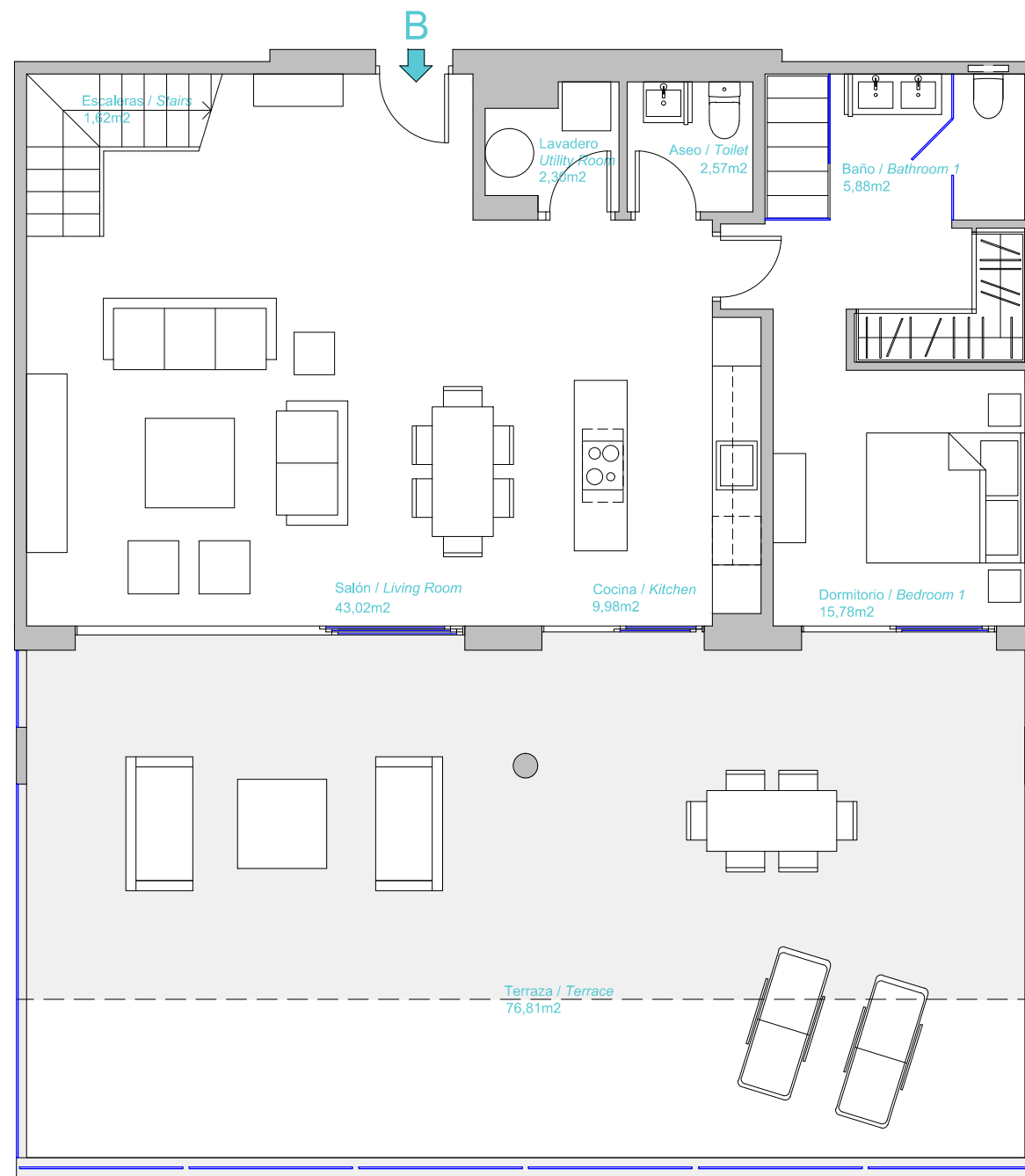
Planta Inferior / Lower Floor
